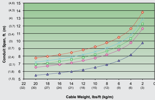
2 ½" (63 mm) SW Conduit (IPS & ID)
