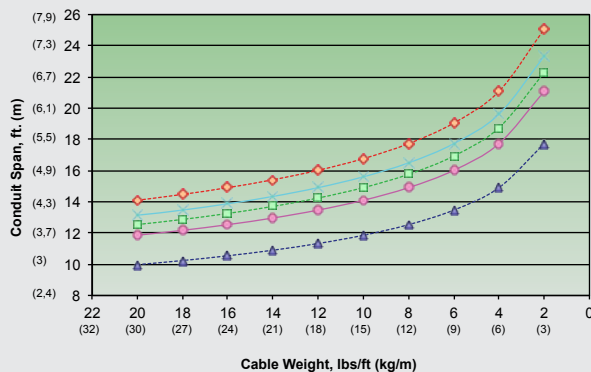
5" (129 mm) HW Conduit (IPS & ID)
